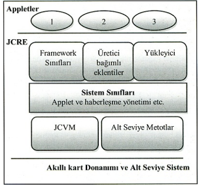
Şekil 3. Java Card Çalışma Zamanı Ortamı
