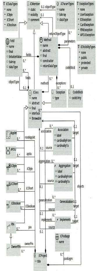
Şekil 4. Java Card API'ye bağlı olarak türetilen Java Card Metamodeli
